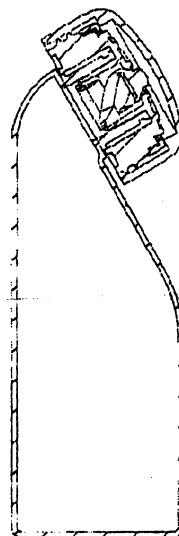
【A-A線部断面図】
