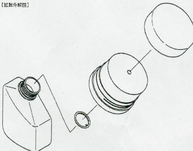
【拡散分解図】
