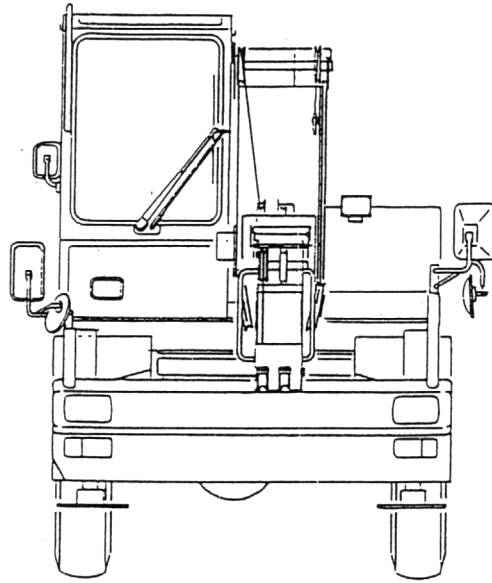
左側面図
