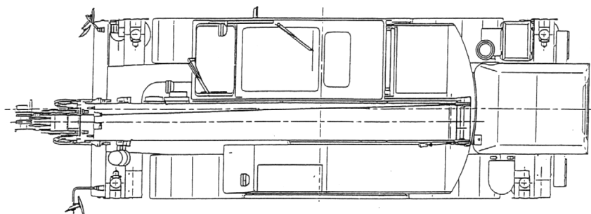
平面图
