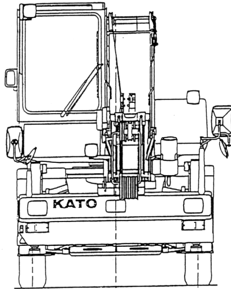
左側面図
